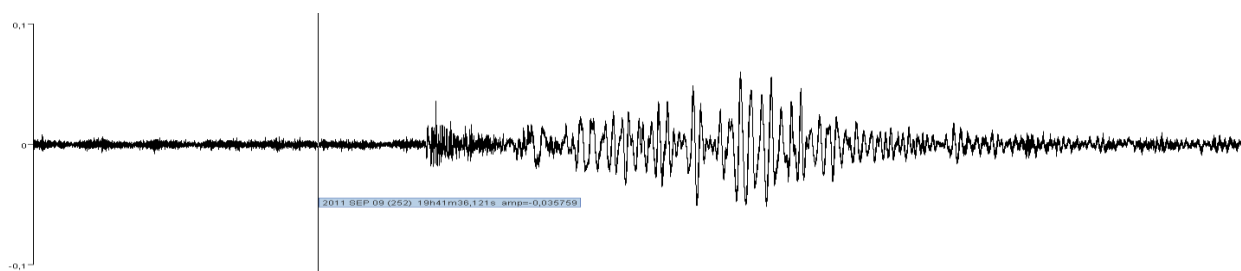
Séisme sur l'île de Vancouver le 9 septembre 2011, enregistré par la toute nouvelle station sismo du lycée français de San Francisco (FRCO)
